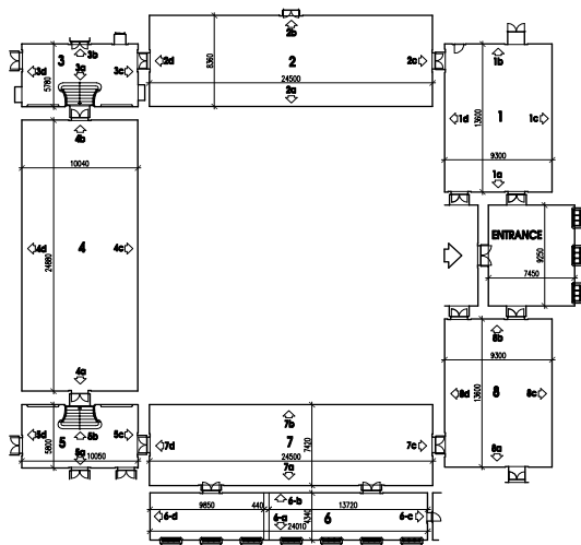
Galerie Rudolfinum - 1. patro - 1:250
