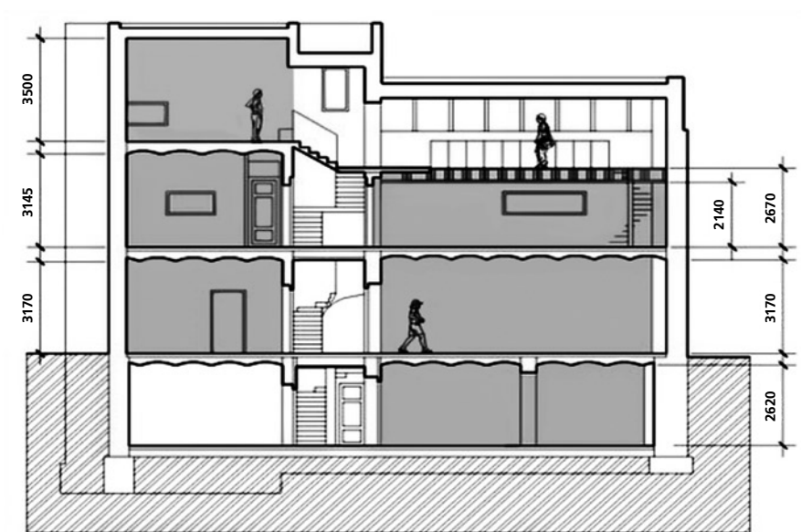
Galerie Langhans - průřez budovou
